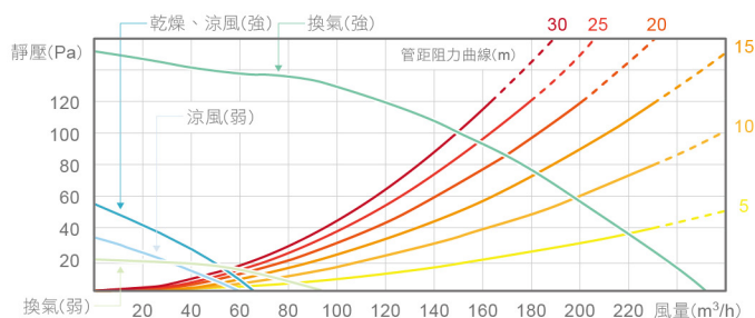
TYB3131AD(110V) 靜壓風量特性曲線
