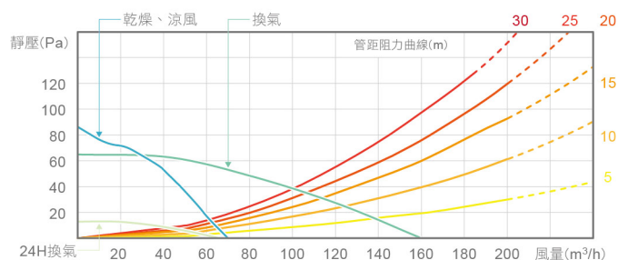
TYB251GKT(220V) 靜壓風量特性曲線
