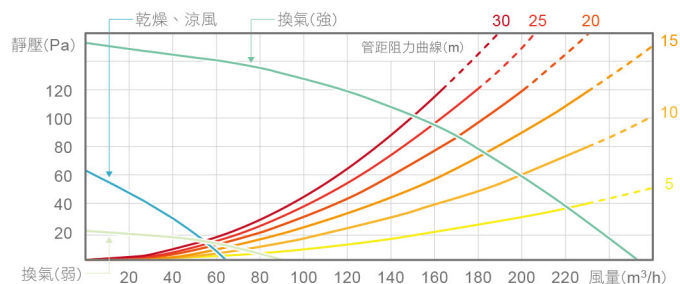
TYB3151AA(220V) 靜壓風量特性曲線
