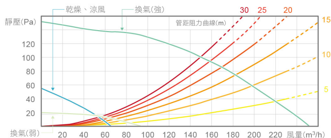
TYB3131AA(110V) 靜壓風量特性曲線
