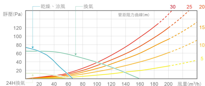
TYB231GKT(110V) 靜壓風量特性曲線
