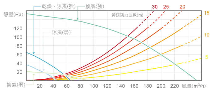
TYB3151AD(220V) 靜壓風量特性曲線
